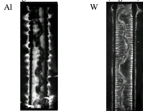
Fig. 10. Schlieren images of 2 wire pinches.
