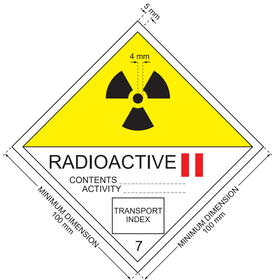
РИС. 3. Знак опасности категории II-ЖЕЛТАЯ (II-YELLOW). Минимальная ширина линии внутри кромки, образующей ромб, – 2 мм. Цвет фона верхней половины знака – желтый, нижней половины – белый, цвет основного знака радиационной опасности (трилистника) и надписей – черный, цвет полос, обозначающих категорию, – красный.
