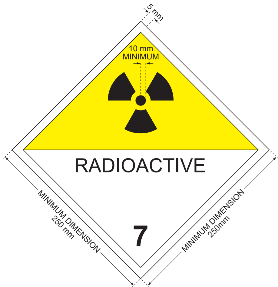
РИС.6. Информационное табло. За исключением случаев, оговоренных в пункте 571, минимальные размеры должны соответствовать размерам, указанным на рисунке; при использовании других размеров должны сохраняться соответствующие пропорции. Высота цифры «7» должна быть не менее 25 мм. Цвет фона верхней половины табло – желтый, нижней половины – белый, цвет основного знака радиационной опасности (трилистника) и надписей – черный. Использование слова «РАДИОАКТИВНО» («RADIOACTIVE») в нижней части не обязательно, что позволяет применять это табло для изображения соответствующего номера ООН для груза.
