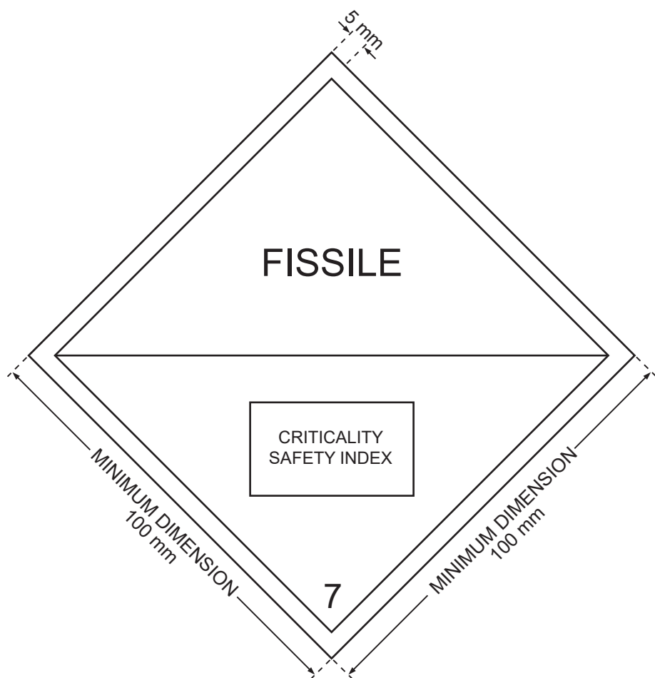
РИС. 5. Знак опасности с указанием ИБК. Минимальная ширина линии внутри кромки, образующей ромб, – 2 мм. Цвет фона знака – белый, цвет надписей – черный.
