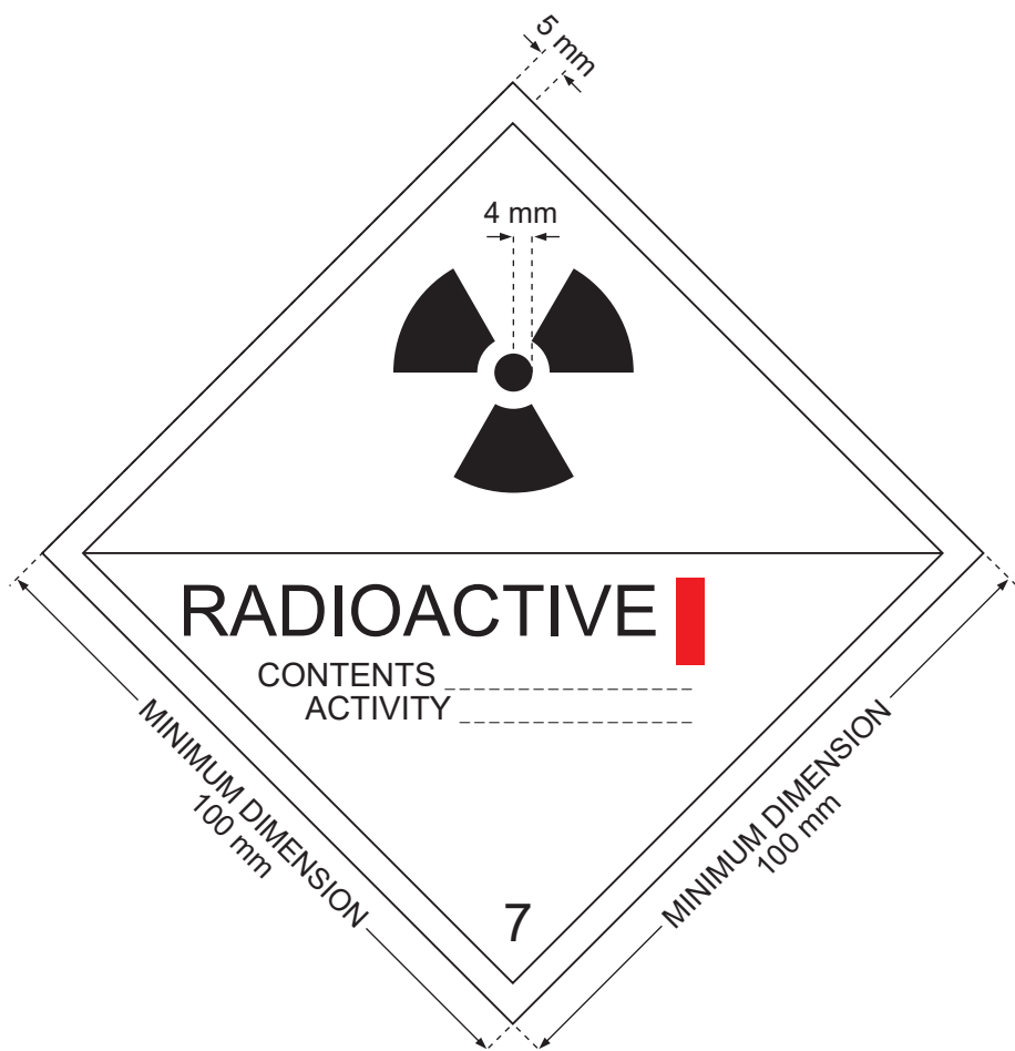
РИС. 2. Знак опасности категории I-БЕЛАЯ (I-WHITE). Минимальная ширина линии внутри кромки, образующей ромб, – 2 мм. Цвет фона знака – белый, цвет основного знака радиационной опасности (трилистника) и надписей – черный, цвет полосы, обозначающей категорию – красный.
