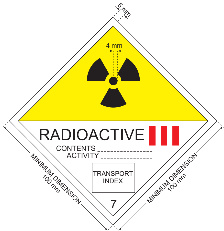
РИС. 4. Знак опасности категории III-ЖЕЛТАЯ (III-YELLOW). Минимальная ширина линии внутри кромки, образующей ромб, – 2 мм. Цвет фона верхней половины знака – желтый, нижней половины – белый, цвет основного знака радиационной опасности (трилистника) и надписей – черный, цвет полос, обозначающих категорию, – красный.
