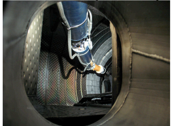
Fig. 2: AIA inside Tore Supra
