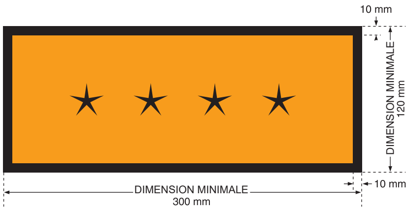
FIG. 7. Placard pour l'affichage séparé du numéro ONU. Le fond du placard est orange, la bordure et le numéro ONU sont noirs. Le symbole « **** » indique l'espace dans lequel le numéro ONU relatif à la matière radioactive (voir le tableau 1) doit être indiqué.
