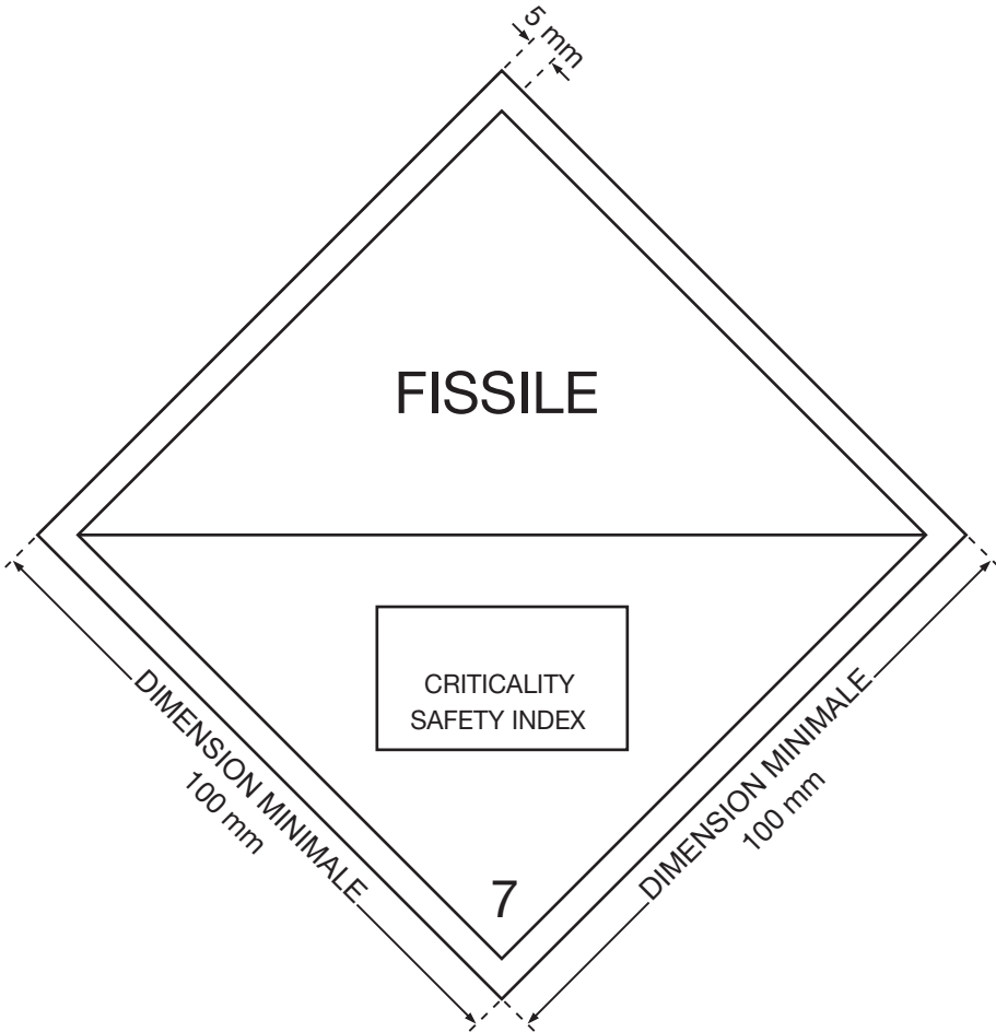
FIG. 5. Étiquette pour le CSI (indice de sûreté-criticité). La largeur minimale de la ligne située à l'intérieur du bord formant le losange doit être de 2 mm. Le fond de l'étiquette est blanc, le texte est noir.
